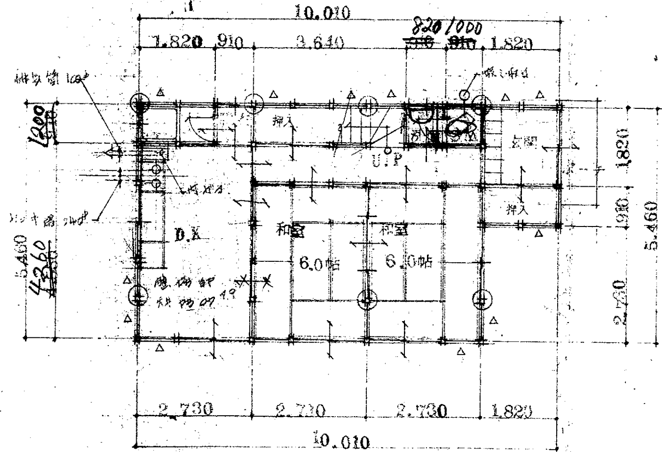
1層 平面图 S:1/100
