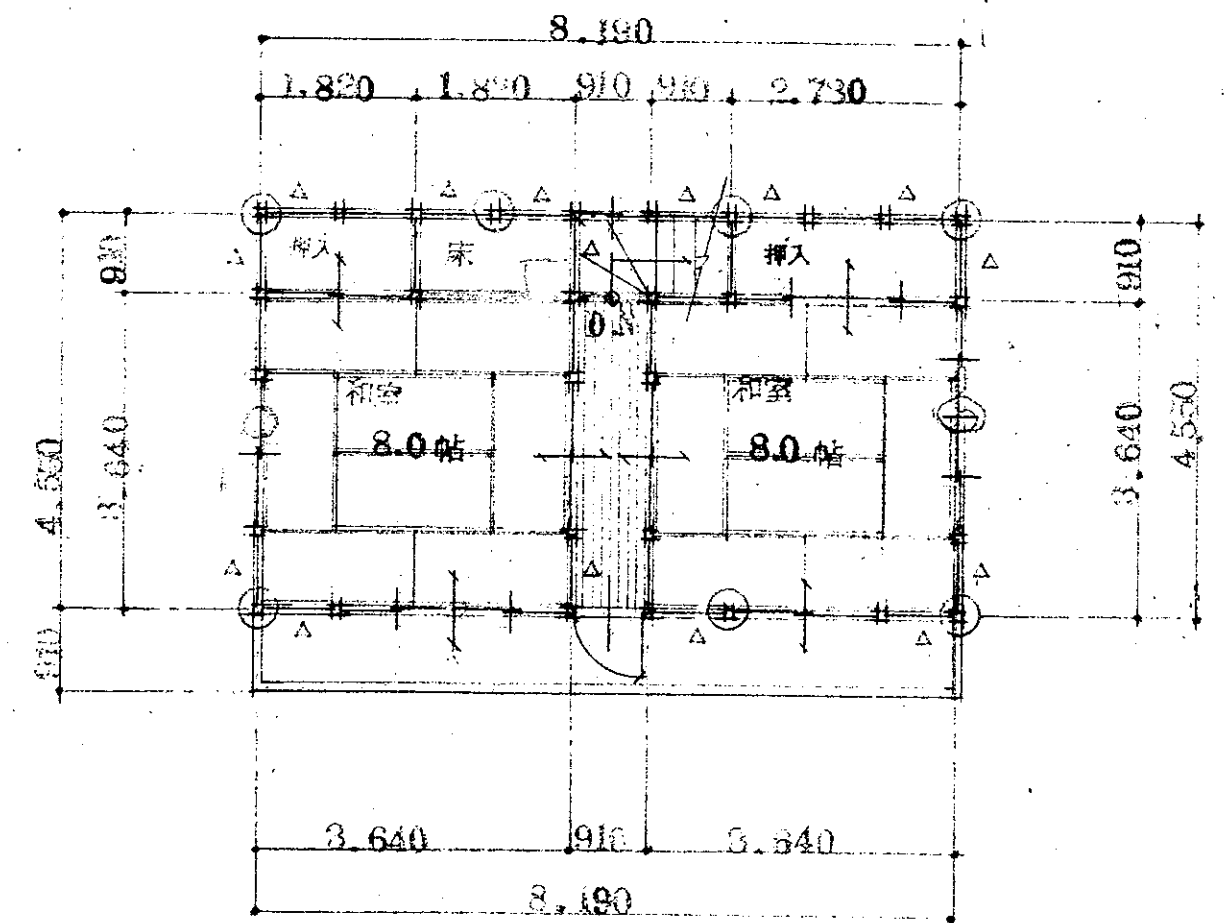
2層 平面图 S:1/100
